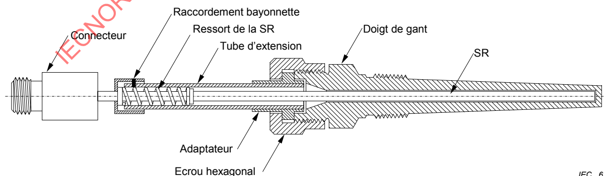
Figure 1 – Forme et dimensions d'une SR
