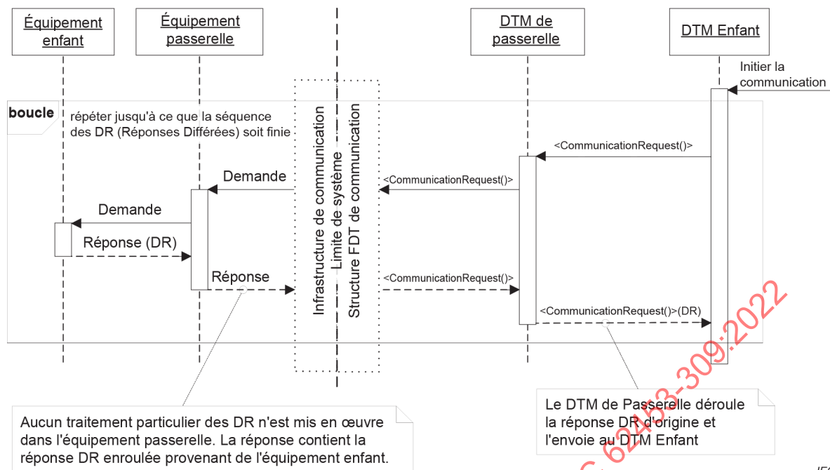
Figure 3 – Traitement des réponses différées (scénario 1)
