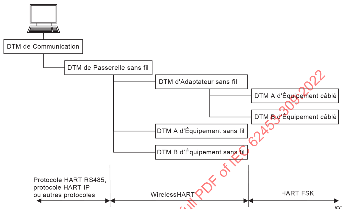
Figure 8 – Topologie FDT d'un réseau WirelessHART
