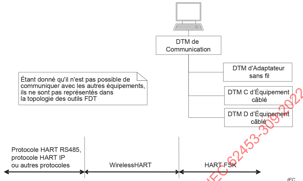
Figure 10 – Topologie FDT dans le cas d'une connexion directe à un équipement adaptateur WirelessHART
