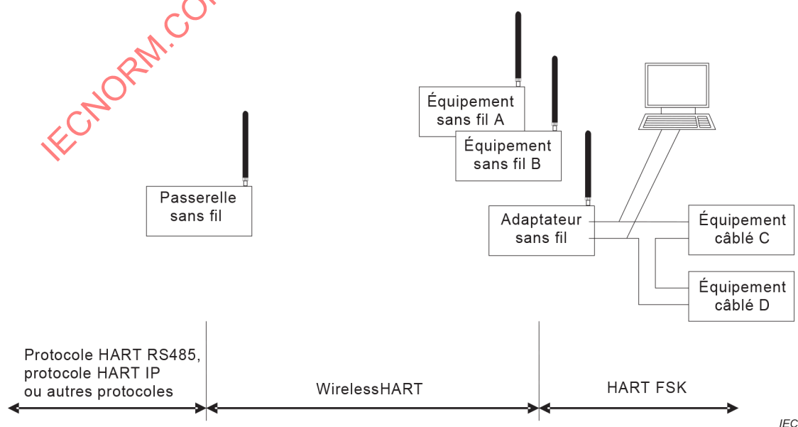
Figure 9 – Hôte connecté à HART FSK
