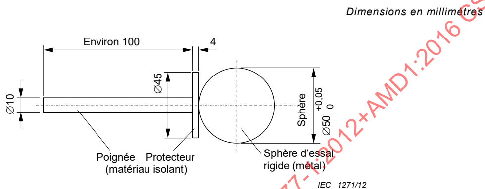
Figure M.1 – Sphère d'essai de 50 mm (IPXXA)
