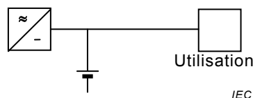
Figure 3 – Fonctionnement en mode parallèle (y compris modes de fonctionnement de secours et tampon)
