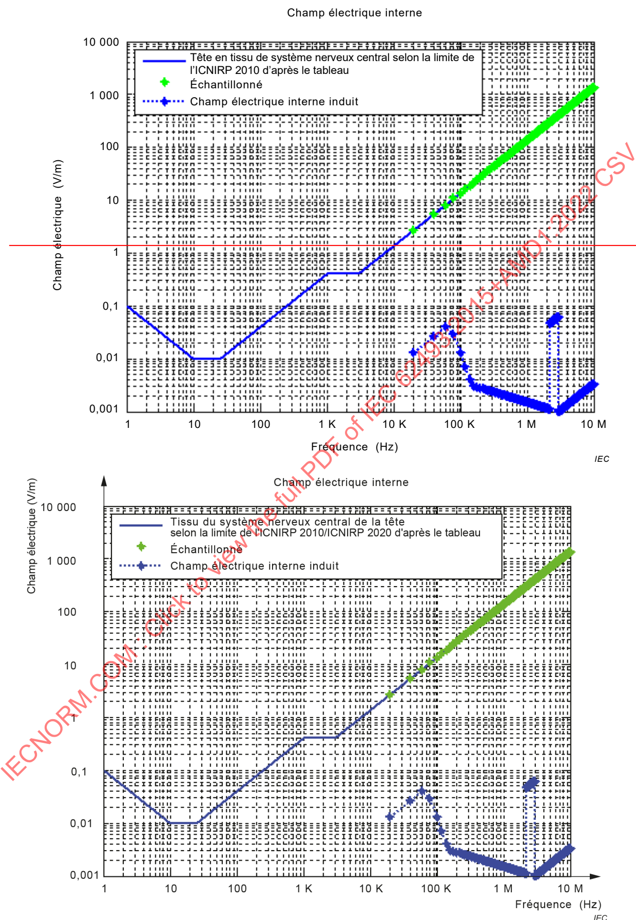
Figure D.4 – Champ électrique interne induit et niveaux limites associés
