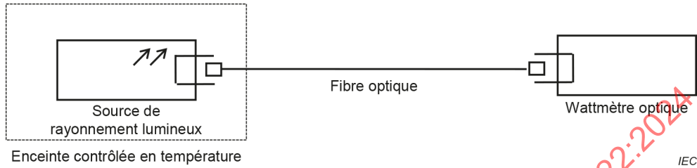
Figure 6 – Montage de mesure de la dépendance par rapport à la température
