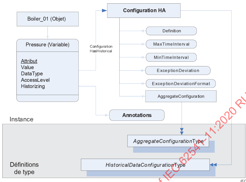
Figure 3 – Variable d'historique avec Configuration et Annotations de données historiques
