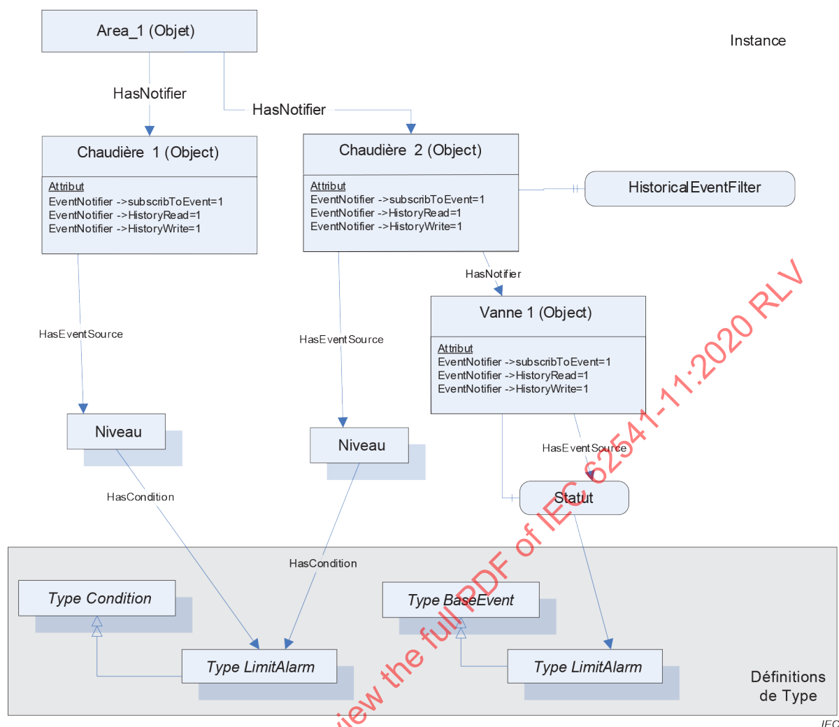
Figure 4 – Représentation d'un Événement à l'aide de l'Historique dans l'AddressSpace
