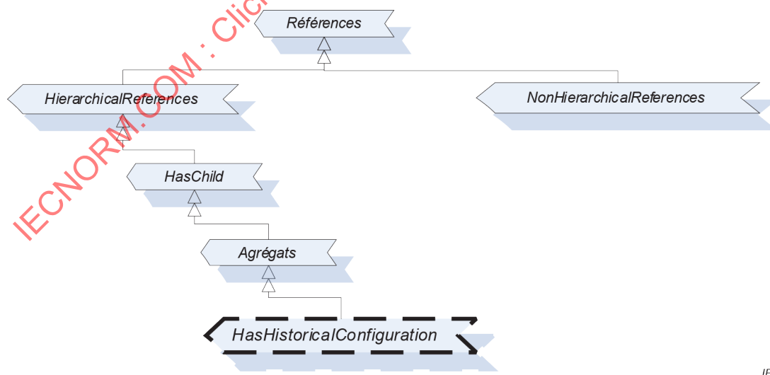
Figure 2 – Hiérarchie de ReferenceType
