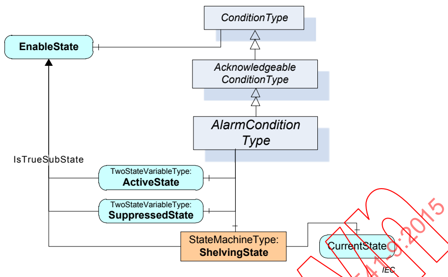
Figure 12 – Modèle Alarm
