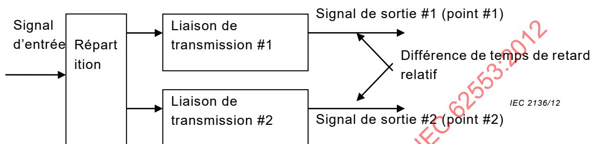
Figure 2 b) – Définition de la différence de temps de retard relatif
