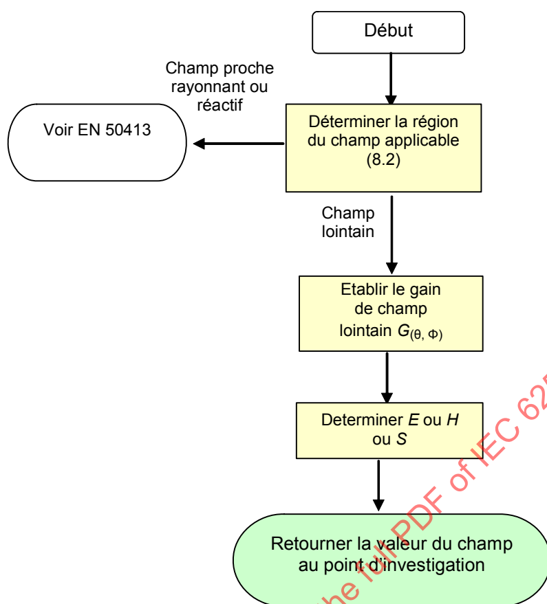
Figure 1 – Procédures alternatives pour calculer les valeurs de champ E , H au point d'investigation
