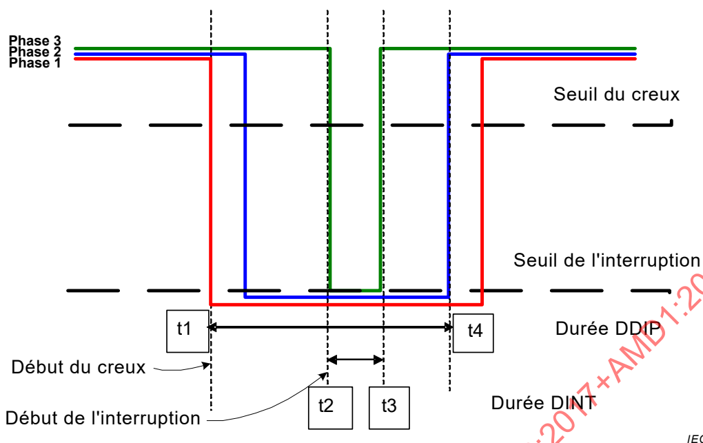
Figure 40 – Détail 1 de la forme d'onde pour l'essai des creux/coupures polyphasés
