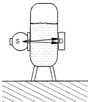
Jauge de niveau fixe ou de densité
