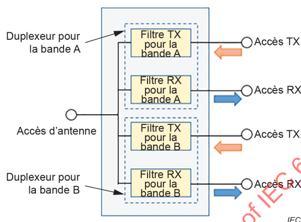
a) Combinaison de deux duplexeurs
