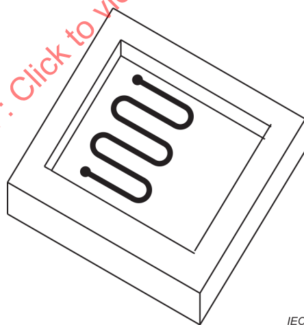
Figure 13 – Déphaseur par ligne à microruban sur la surface d'un boîtier en céramique
