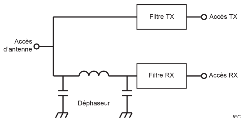
Figure 14 – Déphaseur à éléments localisés
