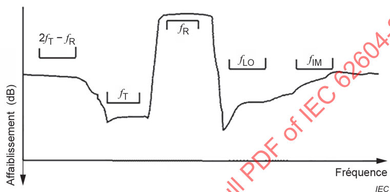
Figure 12 – Réponse en fréquence à large bande type du filtre RX pour le système local supérieur
