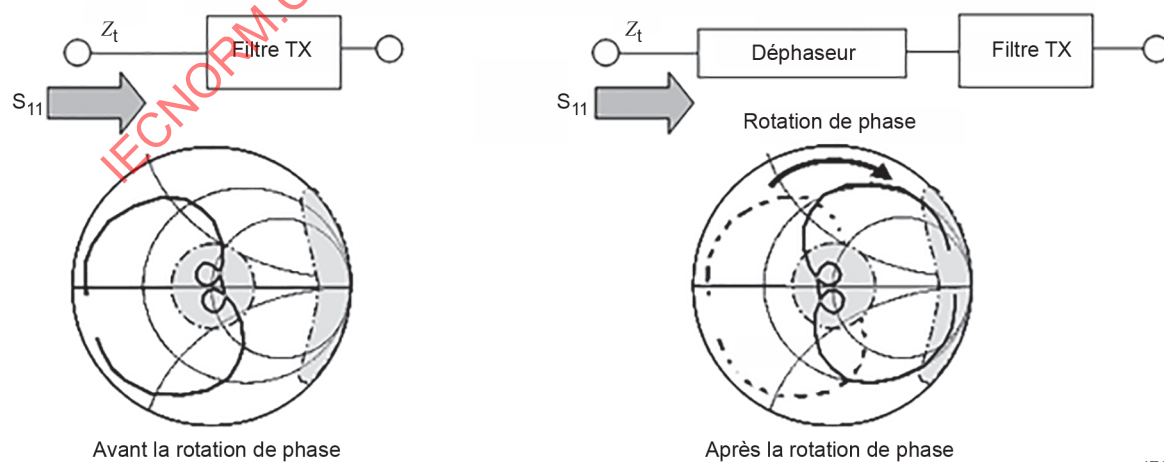
Figure 7 – Rotation de phase dans la partie TX
