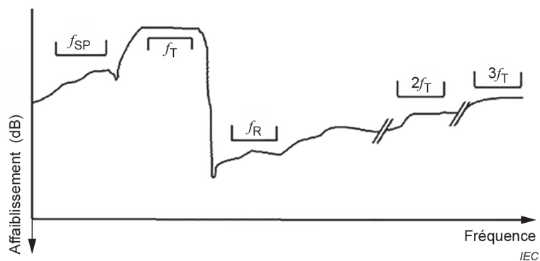
Figure 11 – Réponse en fréquence à large bande type du filtre TX
