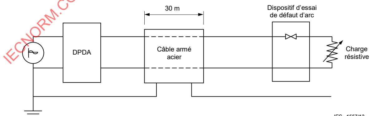
Figure 14 – Description du filtre IEM décrit en Figure 13
