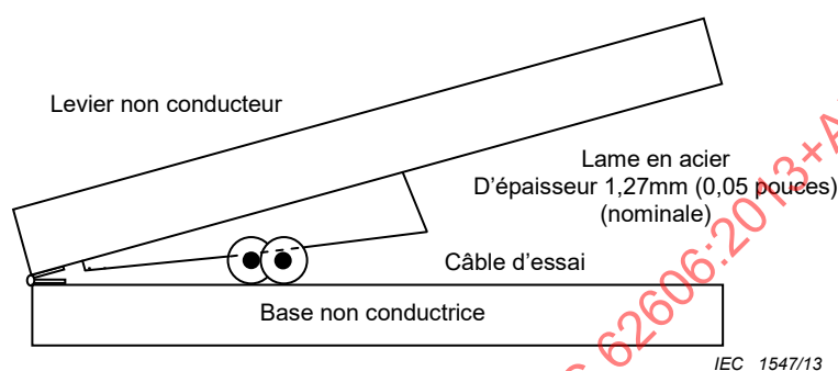
Figure 8 – Appareil d'essai
