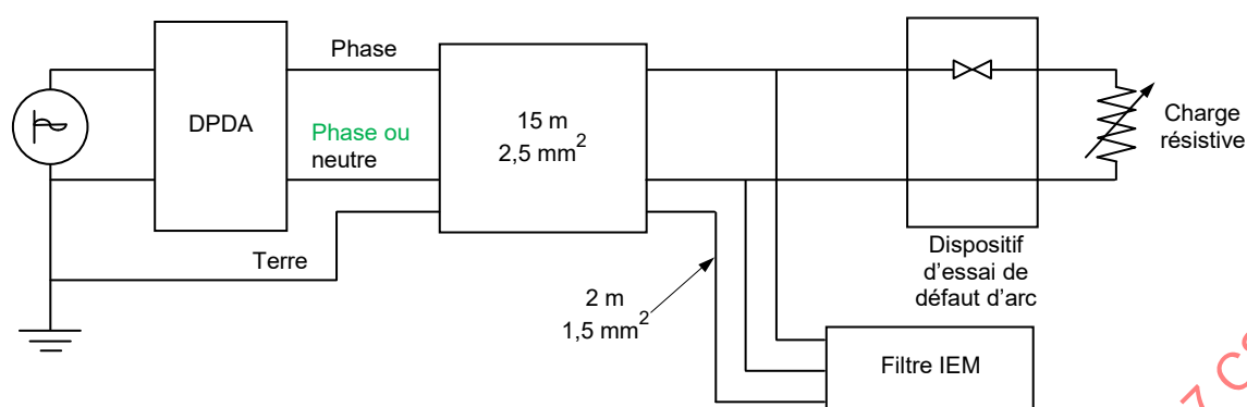
Figure 13 – Filtre IEM 2 pour essais de masquage
