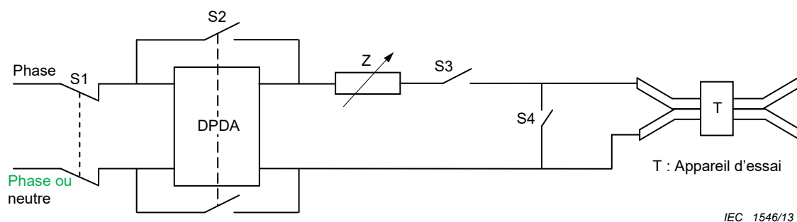
Figure 7 – Circuit d'essai en cas d'arc parallèle et d'essai de coupure de câble
