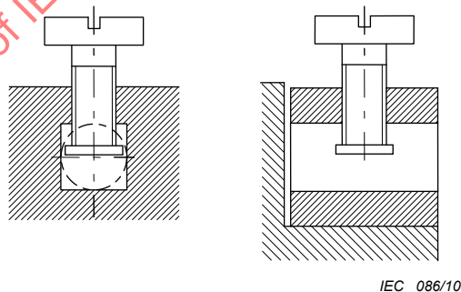
Figure IB.1c – Bornes avec plaquette
