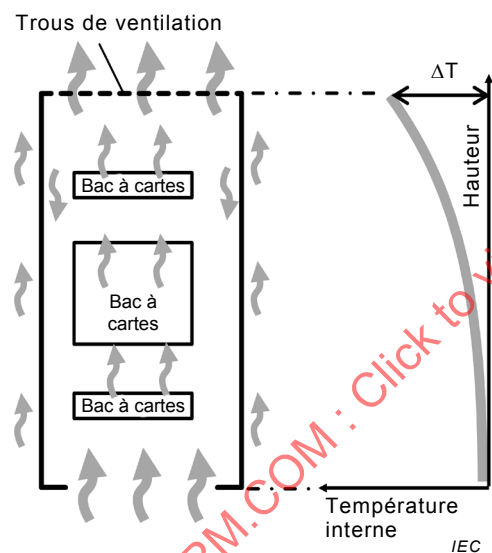
Figure 2a – Baie non scellée sans dispositifs de circulation d'air – ventilée
