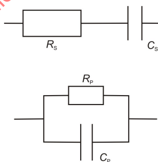
Figure 2 – Schémas de circuits équivalents
