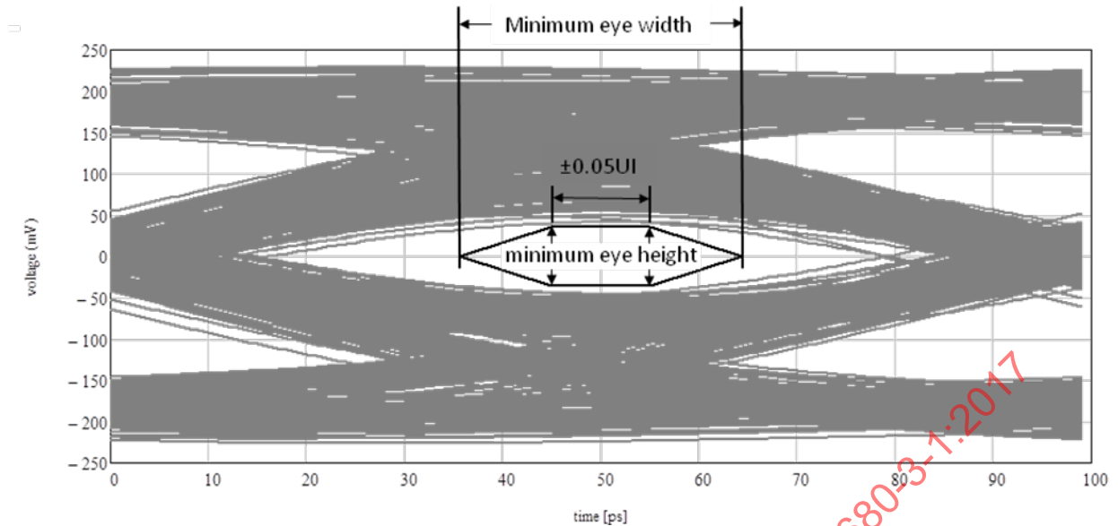
Gen 2 eye mask
