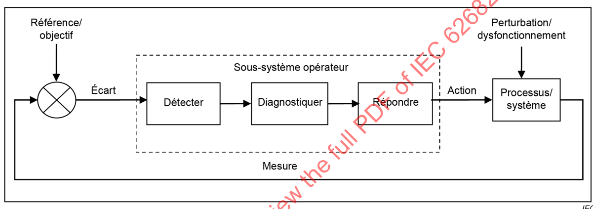
Figure 5 – Modèle de rétroaction de l'interaction opérateur-processus
