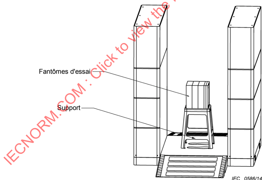
Figure 1 – Illustration générique de la configuration d'essai montrant un fantôme corps en PEHD avec un objet d'essai sur une extrémité supporté à 1 m du sol
