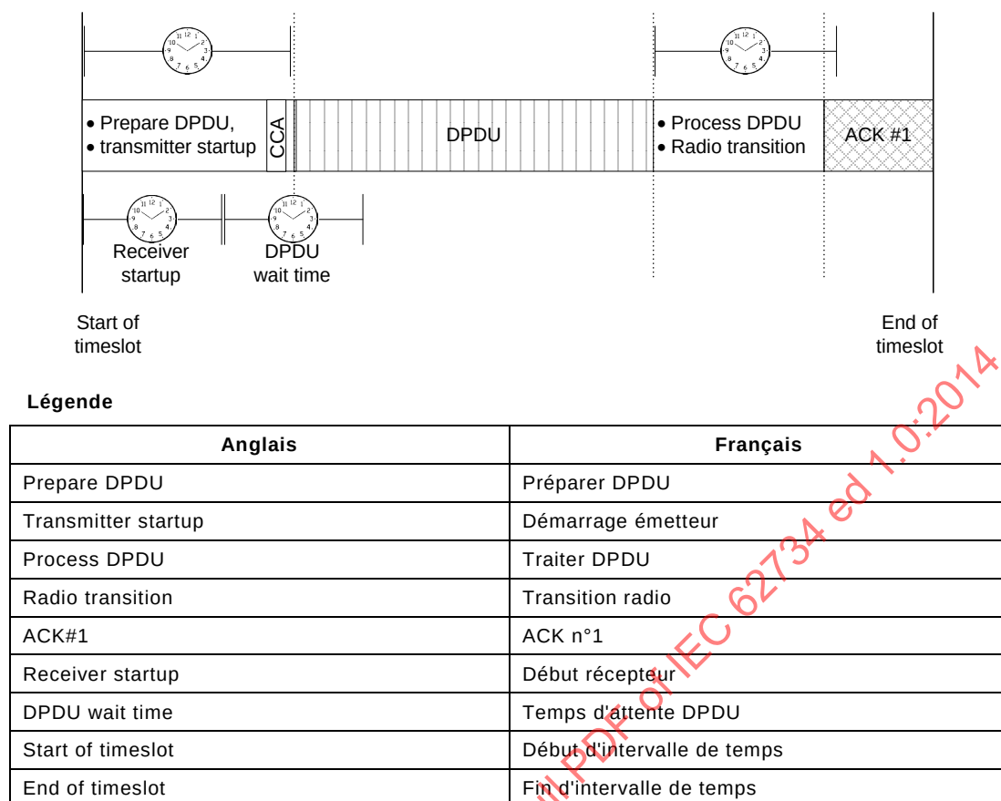
Figure 79 – Attributs de temporisation de transaction
