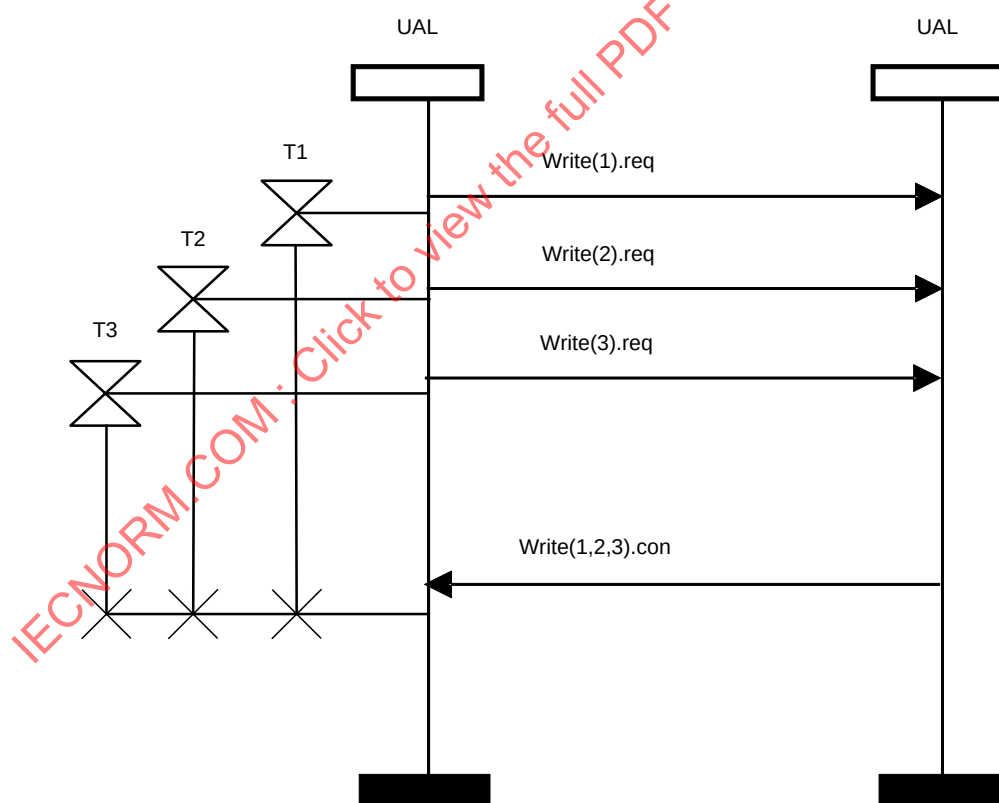
Figure 113 – Exemple réussi de plusieurs demandes en cours avec concaténation des réponses
