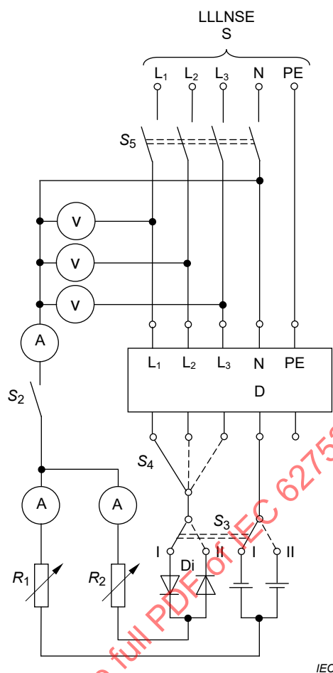
Figure 11c) – Type LLLNSE/LLLNE
