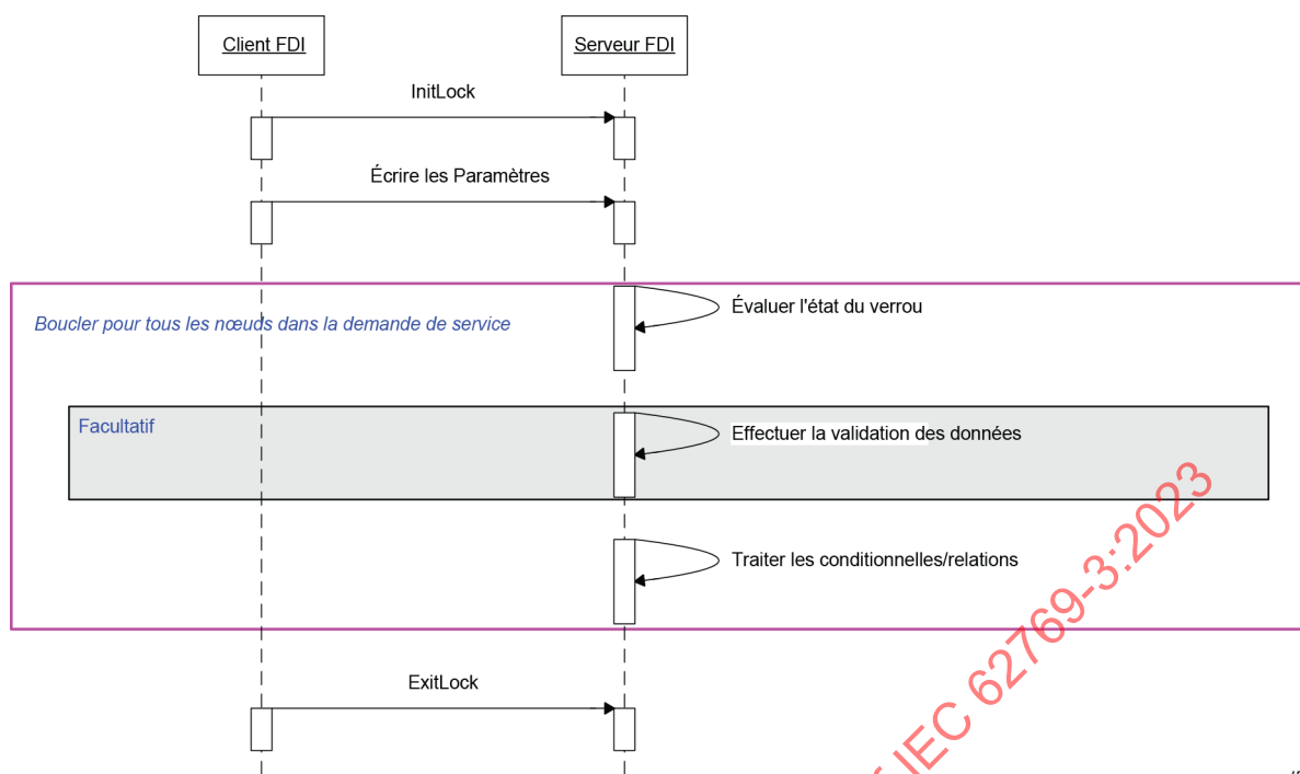
Figure 9 – Ecriture immédiate de variables hors-ligne
