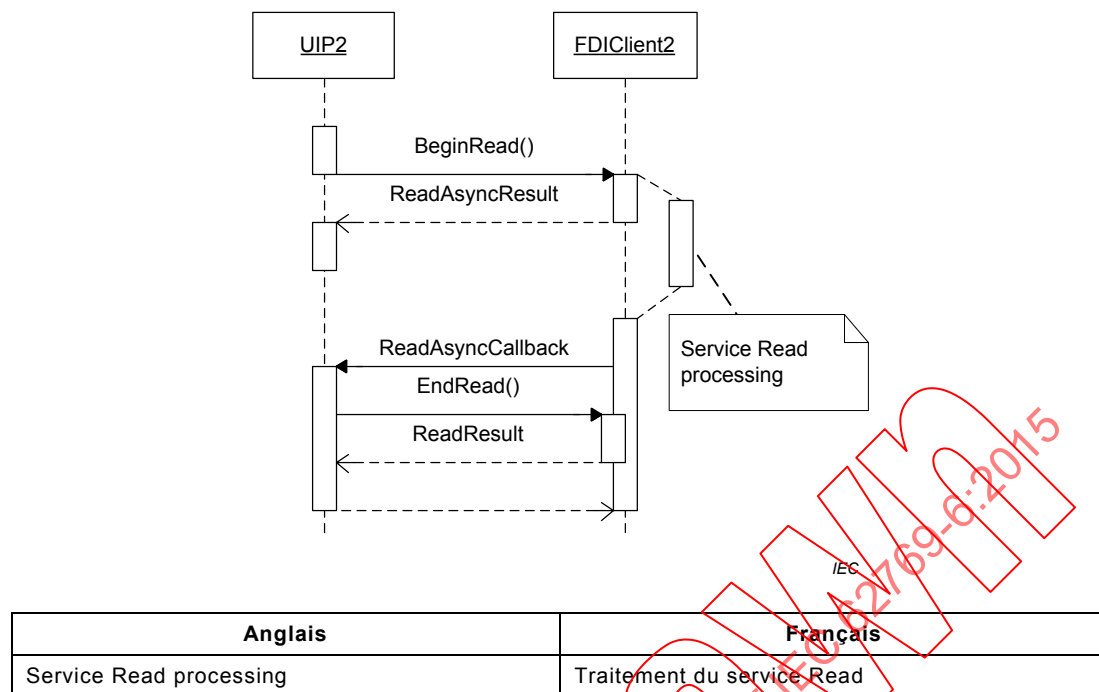
Figure 4 – Exemple d'exécution de service asynchrone basé sur IAsyncResultPattern
