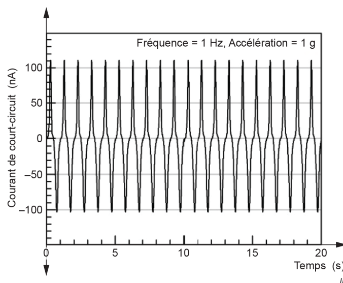
Figure 6 – Courant de court-circuit d'un récupérateur d'énergie piézoélectrique souple
