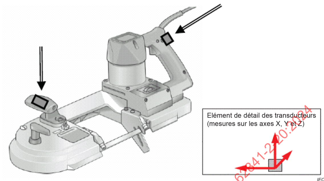
Figure I.101 – Positions des transducteurs pour les scies à ruban
