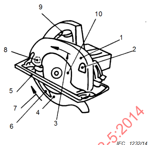
Figure 102 – Scie circulaire à protecteur pendulaire intérieur
