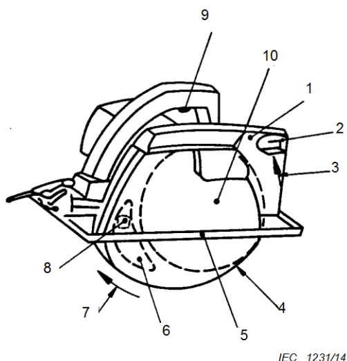
Figure 101 – Scie circulaire à protecteur pendulaire extérieur
