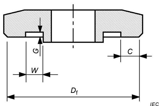
a) Exemple a) de conception de flasque
