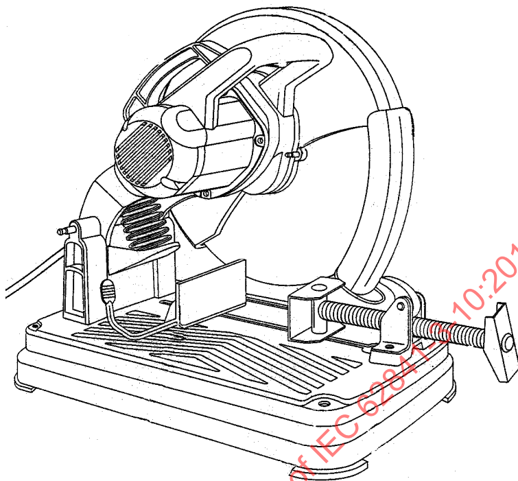
Figure 101 – Exemple de tronçonneuse à disque
