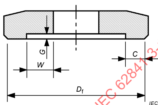
b) Exemple b) de conception de flasque
