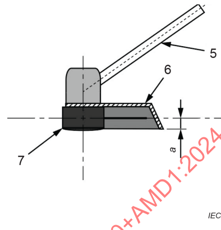
b) View A-A
