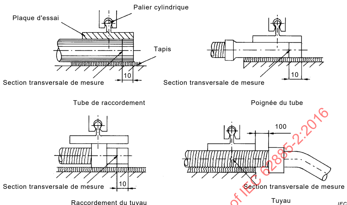
Figure 13 – Position de l'objet d'essai et section transversale de mesure de la déformation
