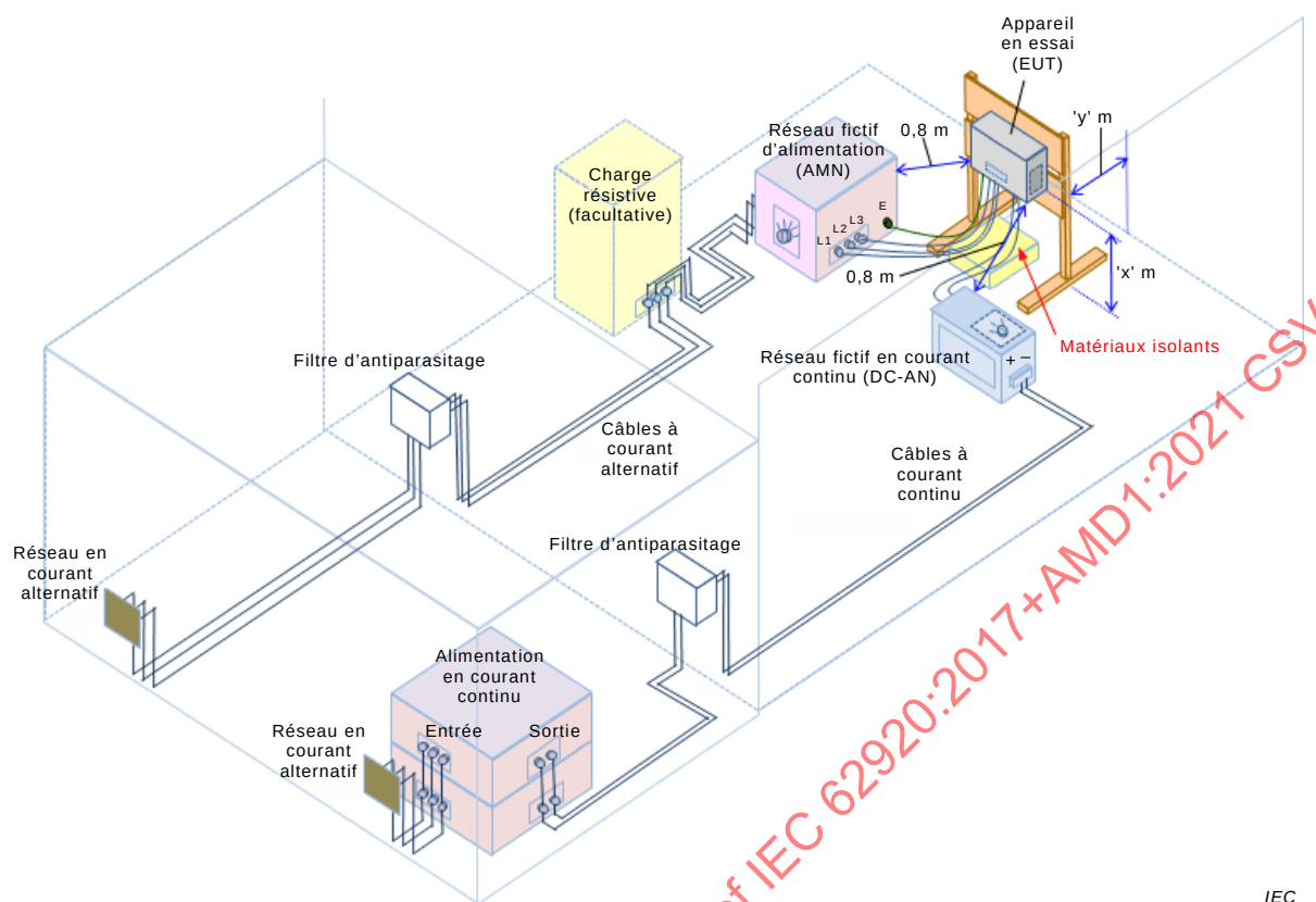
Figure A.12 – Exemple de montage d'essai pour le mesurage des perturbations conduites appliqué à un PCE fixé au mur avec connexion directe au réseau en courant alternatif
