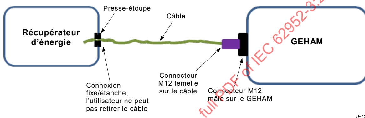
Figure A.1 – Option 1: Connexion fixe à un récupérateur d'énergie, connecteur relié au GEHAM
