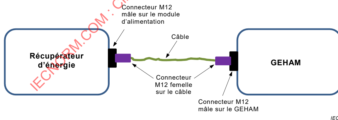
Figure A.2 – Option 2: Connecteurs reliés au récupérateur d'énergie et au GEHAM
