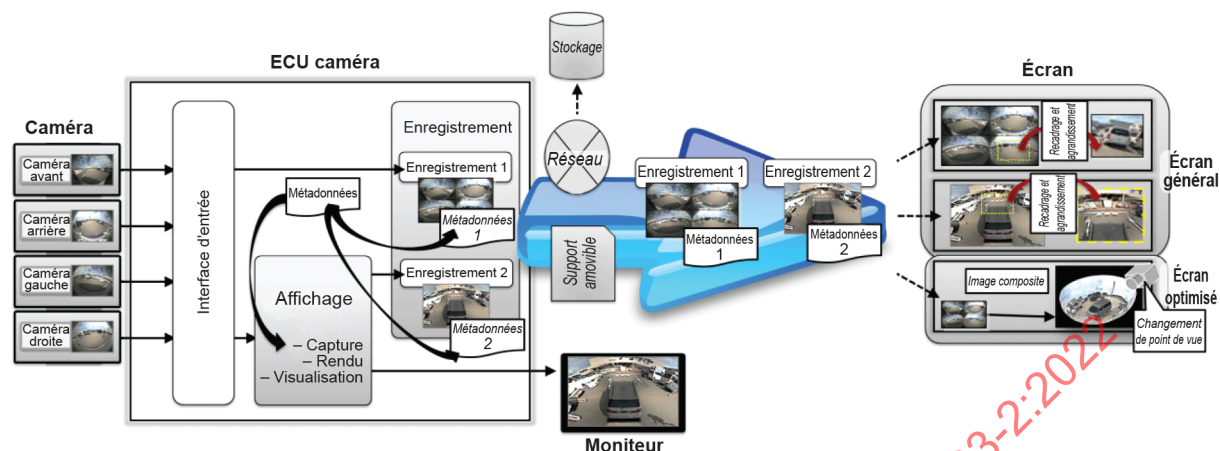
Figure 1 – Modèle du système d'affichage et d'enregistrement du système de vision panoramique
