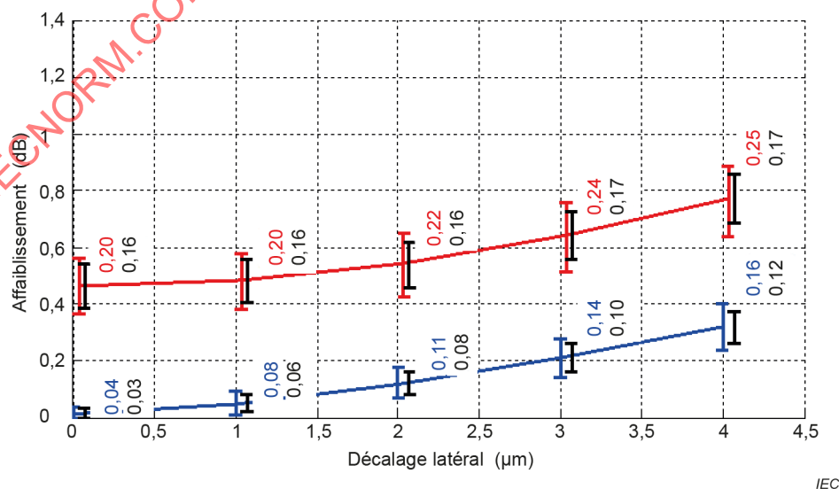
Figure A.1 – Incidence d'incertitude de mesure de l'affaiblissement pour les connexions de référence de classe R_{m1} résultant du décalage latéral et du défaut d'adaptation de l'ouverture numérique (NA) et du diamètre du cœur CD
