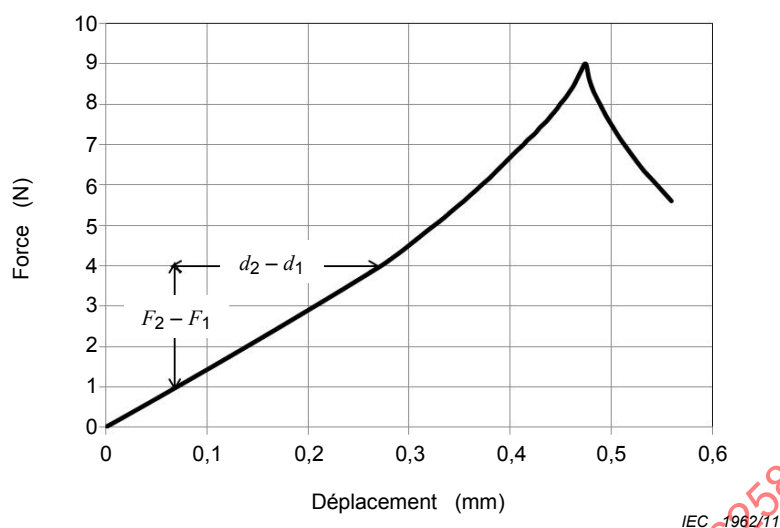
Figure 2 – Calcul du module indenter
