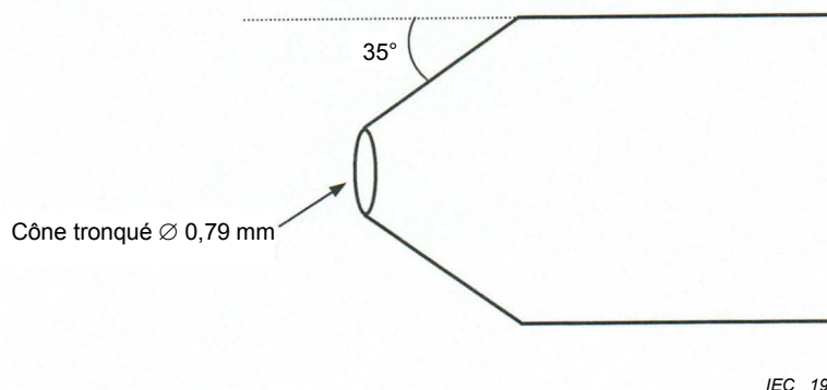
Figure 1 – Représentation schématique de la géométrie et des dimensions de l'extrémité de la sonde utilisée pour le poinçonnement
