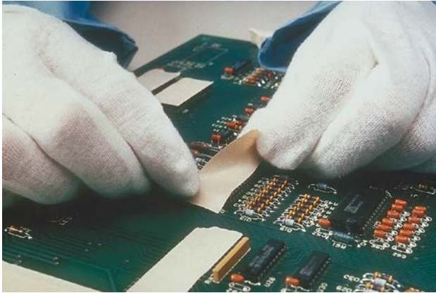
Fig. G3: Manual masking
