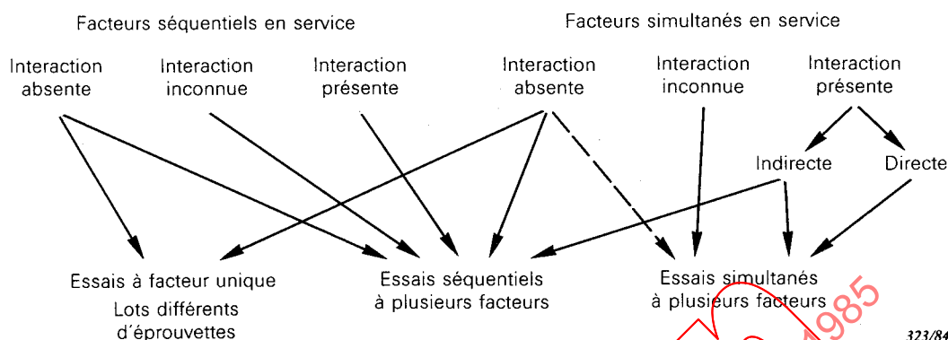
FIG. 1. — Diagramme pour le choix d'une procédure d'essai valable suivant les relations connues ou observées expérimentalement entre facteurs en service.
