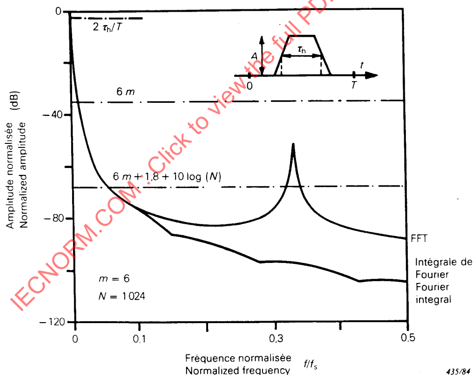
FIG. 9. — Spectre FFT et intégrale de Fourier d'une impulsion trapézoïdale (paragraphe 5.5.2.1c)). FFT-spectrum and Fourier integral of a trapezoidal pulse (Sub-clause 5.5.2.1c)).
