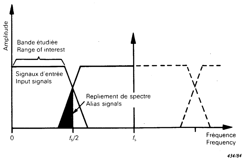
FIG. 8. — Apparition des erreurs d'échantillonnage (paragraphe 5.5.2.1a)). Occurrence of aliasing (Sub-clause 5.5.2.1a)).
