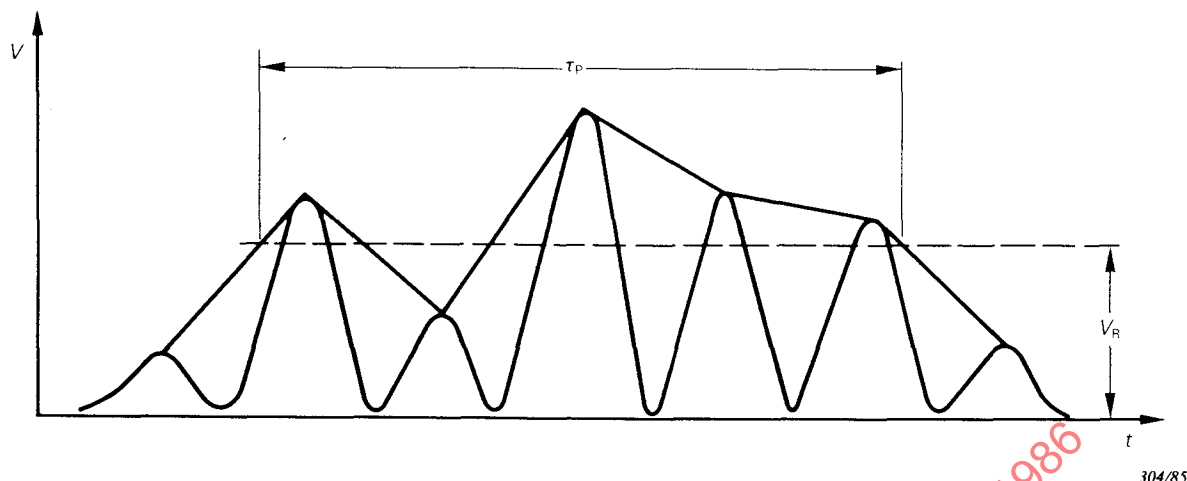
FIG. 1. — Illustration du procédé utilisé pour déterminer la durée \tau_p de l'impulsion réfléchie à partir d'un oscillogramme vidéo de présentation en mode A (paragraphe 8.2). V_R est le niveau de référence d'écho dont il est fait mention dans le texte.
