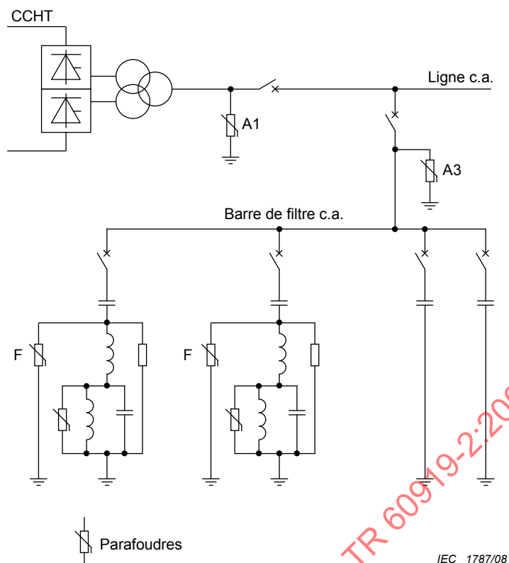
Figure 21 – Exemple de disposition de protection par parafoudre côté c.a. pour une sous-station CCHT
