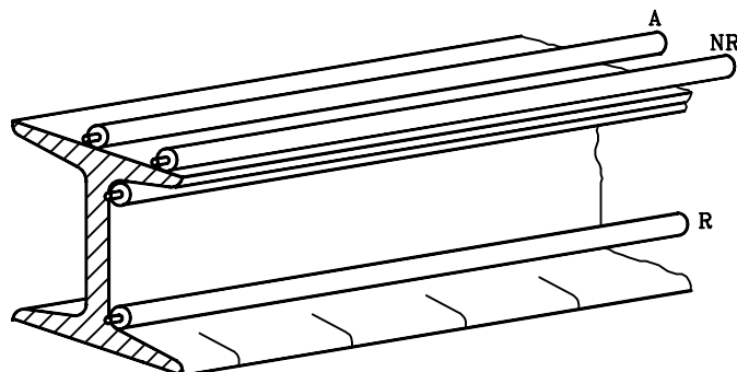
Figure 21 – Position recommandée pour les câbles, parallèlement à une poutre en H, du point de vue de la CEM
