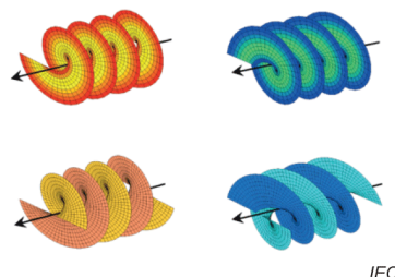
a) LP modes
