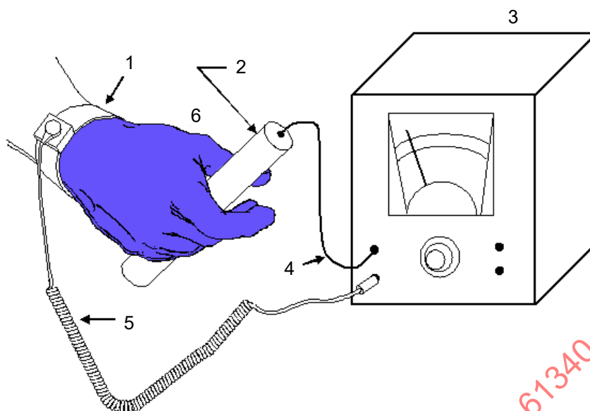
a) – Test using ohmmeter
