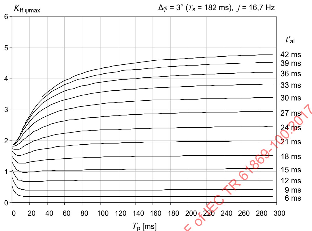
g) T_s = 182 ms at 16,7 Hz
