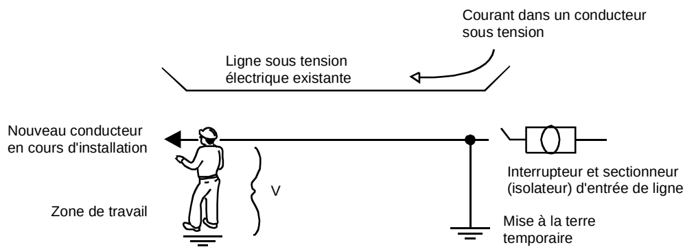
Figure 4a – Tension de circuit ouvert avec une seule terre
