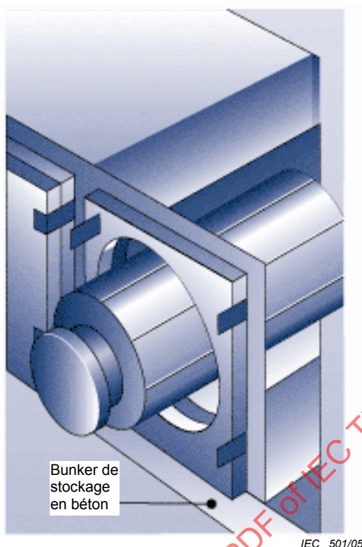
Figure 3 – Chambre horizontale classique d'entreposage de conteneurs de stockage à sec
