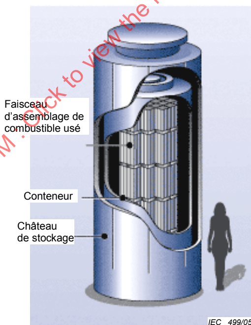
Figure 1 – Château de stockage classique
