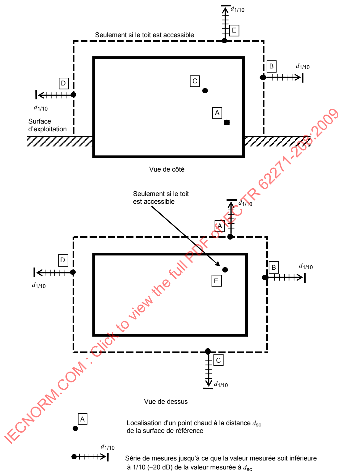
Figure 4 – Détermination des variations de champ en fonction de la distance aux localisations de points chauds (perpendiculairement à la surface de référence)
