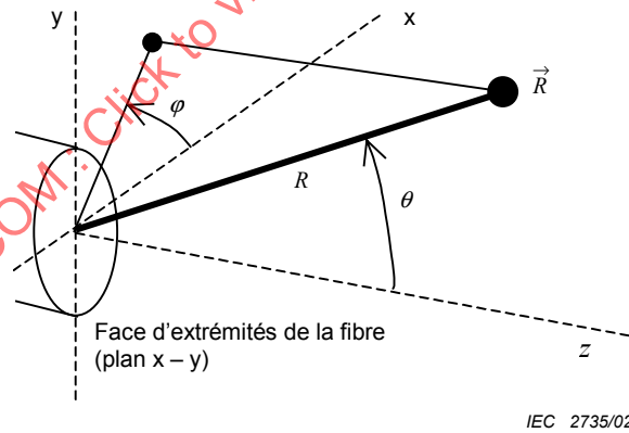
Figure G.2 – Système de coordonnées utilisé pour évaluer le champ de diffraction
