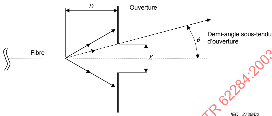
Figure B.2 – Montage de mesure
