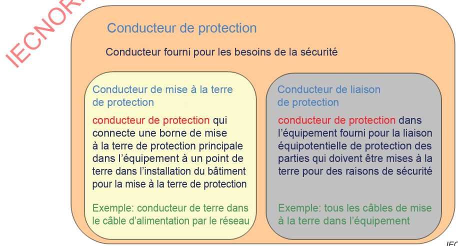
Figure 23 – Aperçu des conducteurs de protection
