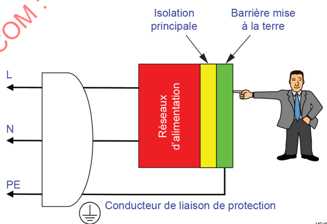
Figure 3 – Conducteur de liaison de protection faisant partie intégrante d'une protection
