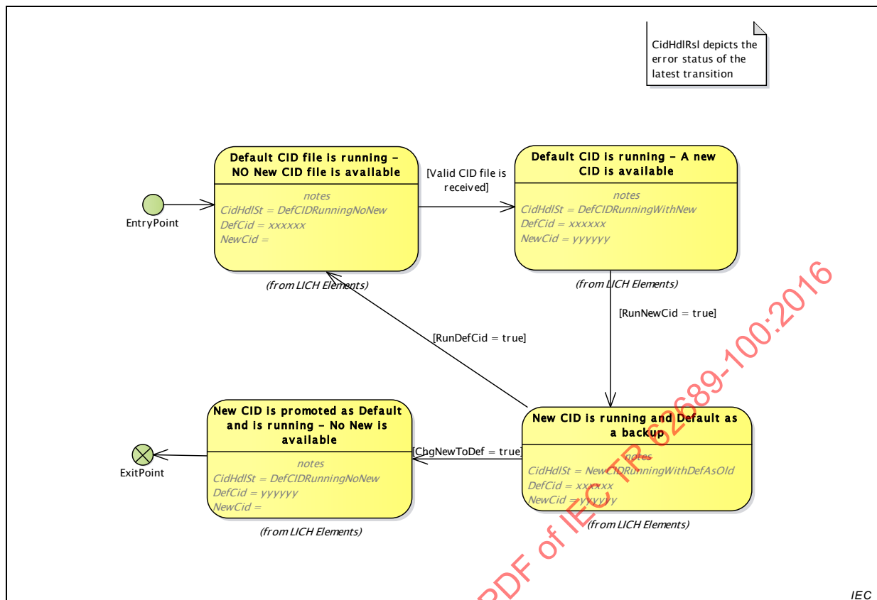
Figure 30 – Statechart diagram LNgrouPL::LNgrouPL
